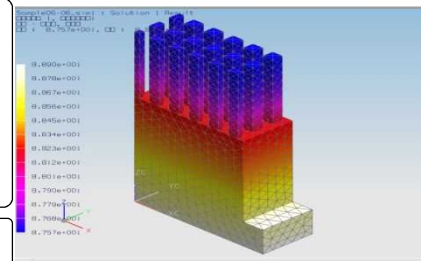
三次元CAD/CAM及びCAEを活用した生産工程の高度化に関する研究 ヒートシンクのCAE解析事例 温度分布 (40.0°C~40.4°C)
